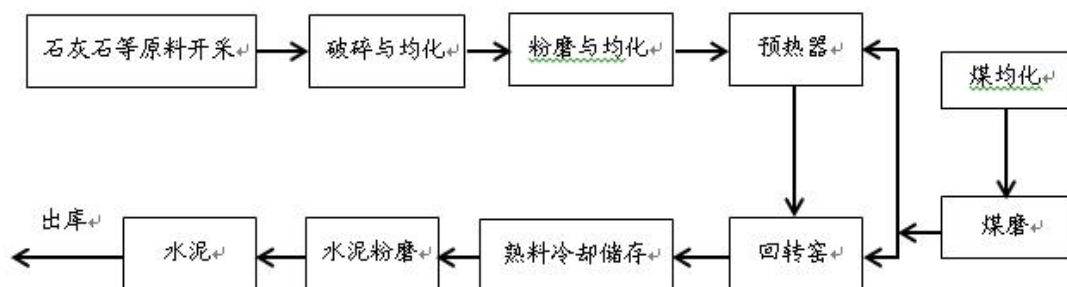
公司水泥生产流程图
